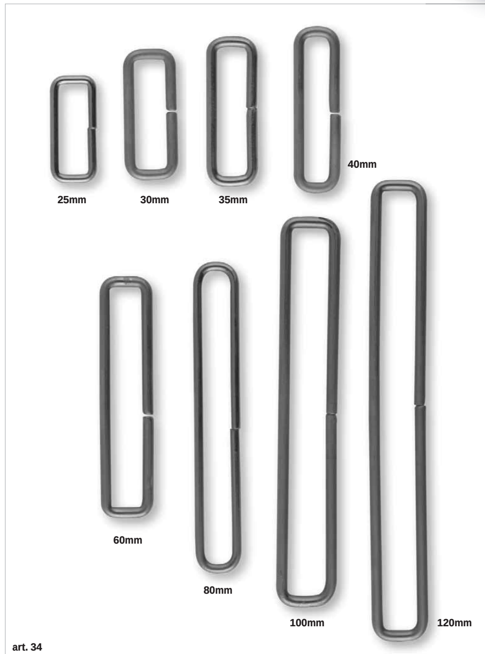
art. 34 PASSANTE in filo tondo rettangolare 25mm-filo 2,5 30mm-filo 3 35mm-filo 3 40mm-filo 3 60mm-filo 3 80mm-filo 2,5 100mm-filo 3 120mm-filo 3
